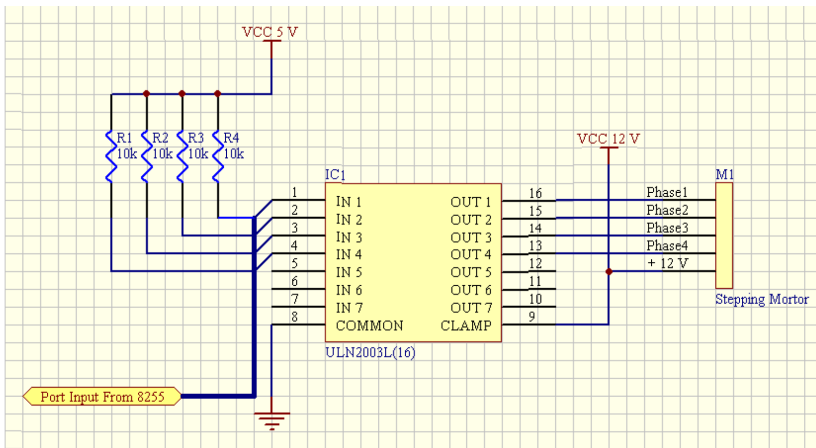
รูปที่ ก.2 รูปแสดงวงจรไดรเวอร์
